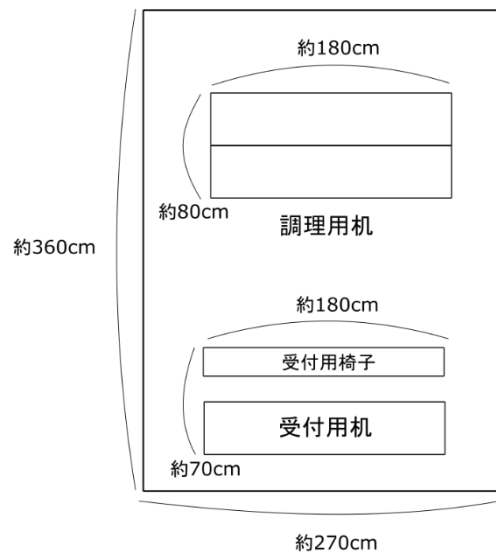
図) 模擬店備品配置例
